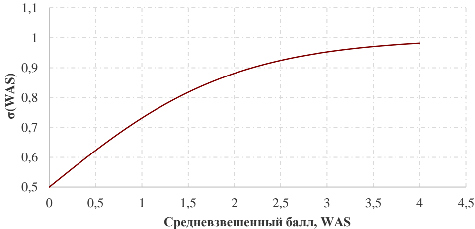
Функция активации сигмоид
